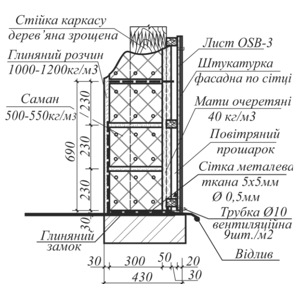
Рис.1. Конструкція стіни житлового будинку з саману
