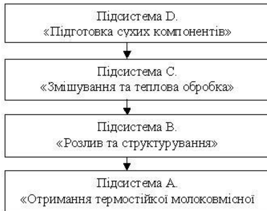
Рисунок – Технологічна система виробництва термостійкої молоковомісної начинки
