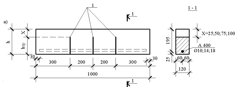
Рис. 1 Експериментальна балка: а) геометричні характеристики; б) розбивка експериментального зразка нормальними тріщинами на окремі блоки; схема армування зразків; 1 - вставка з ДВП
