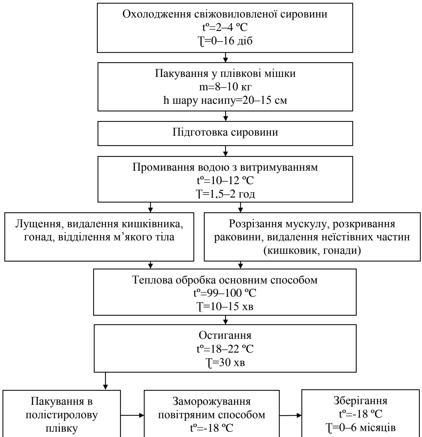
Рис. 1. Технологічна схема виготовлення напівфабрикату з молюска прісноводного
