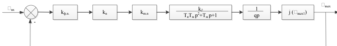
Рис. 2. Вхідна структурна схема
