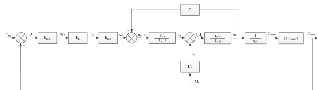
Рис. 2. Вхідна структурна схема
