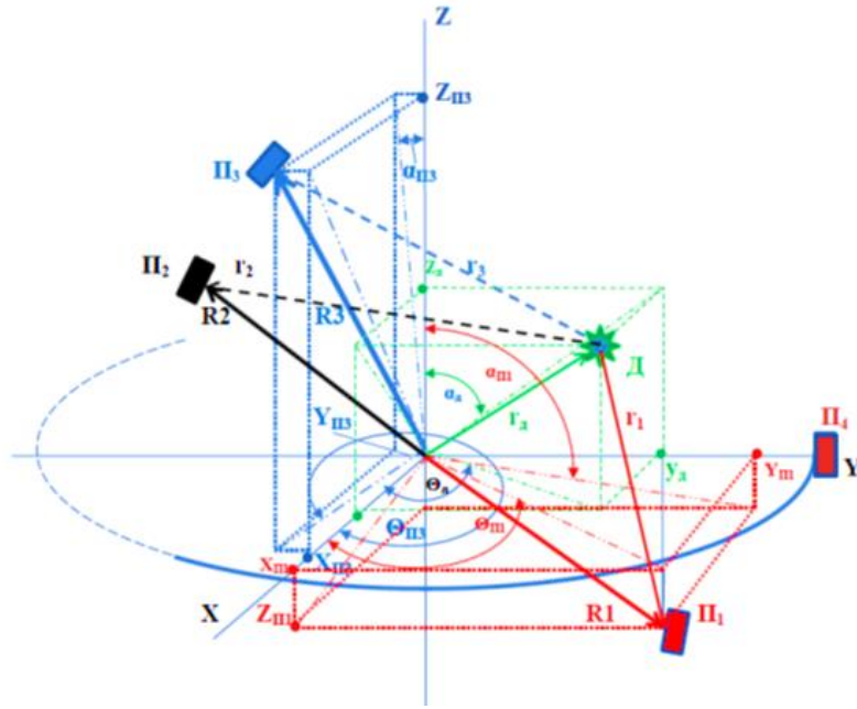
Рисунок 1- Розрахункова модель для визначення координат розташування пошкодження методом ліній положення
