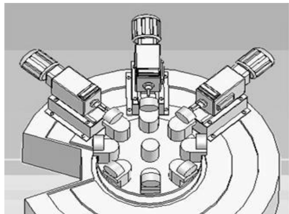
Рис. 8. Компоновка АС из трех горизонтально расположенных силовых агрегатов.
