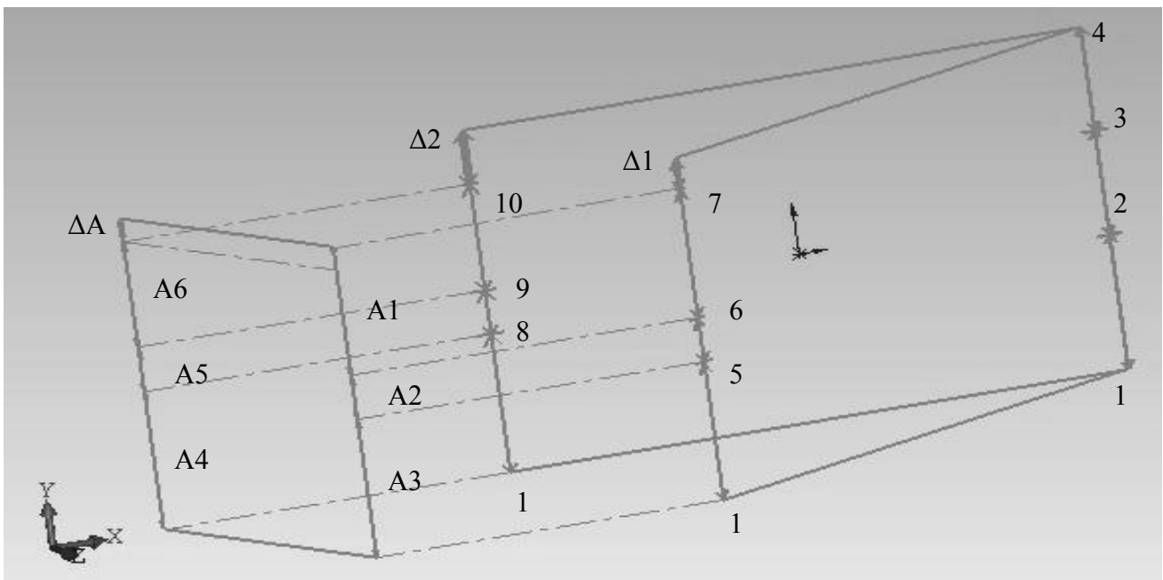
Рис.7. Схема пространственной размерной цепи А.
