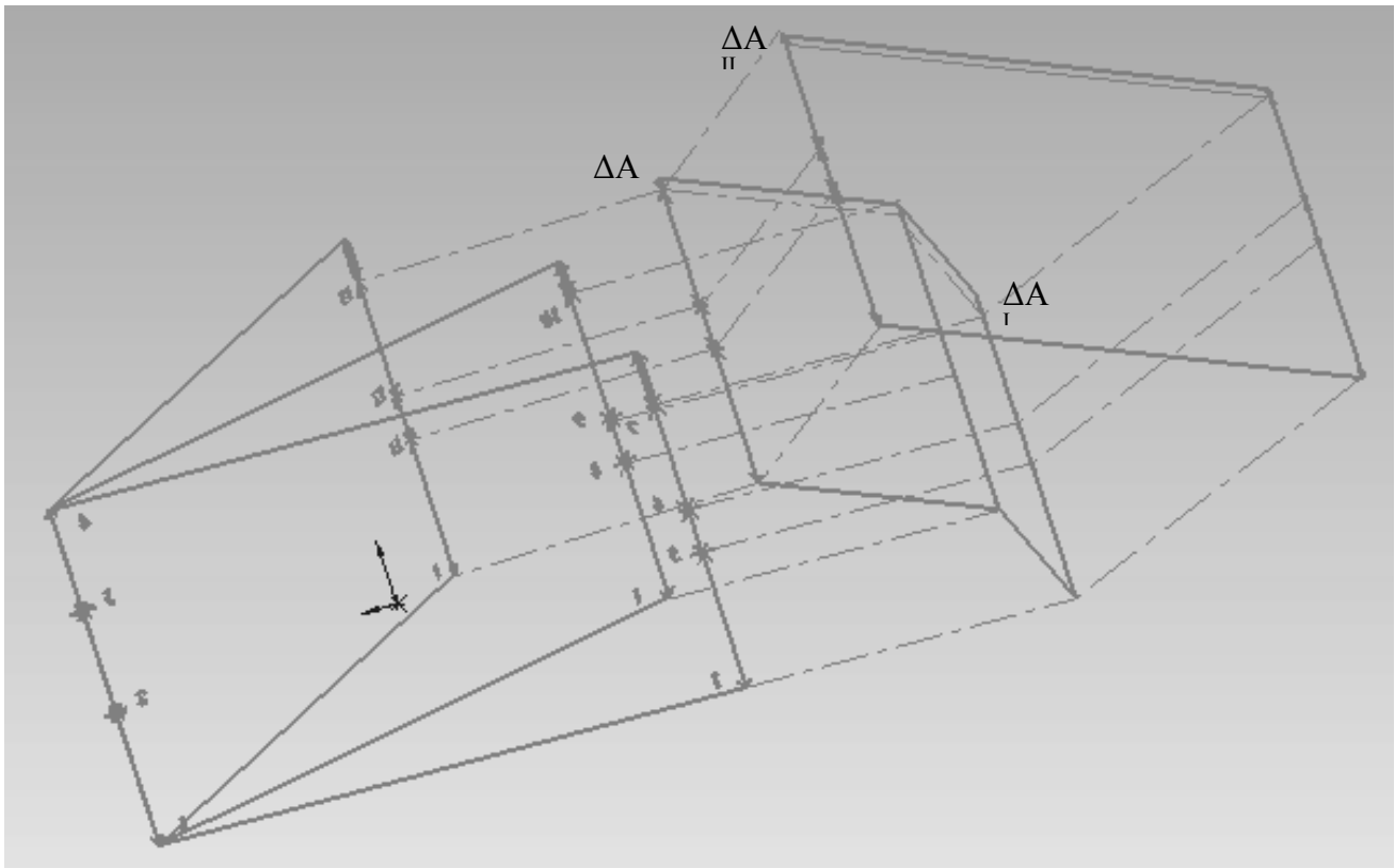
Рис. 9. Пространственная схема размерных цепей.
