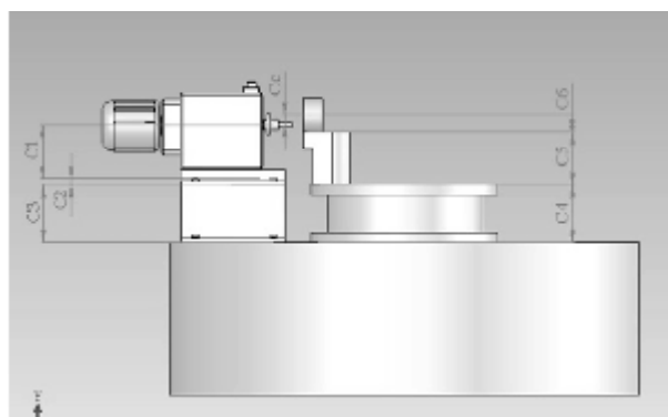
Рис. 1. Модель размерной цепи С.
