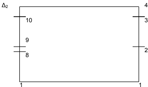
Рис. 4. Схема размерной цепи для второй позиции.
