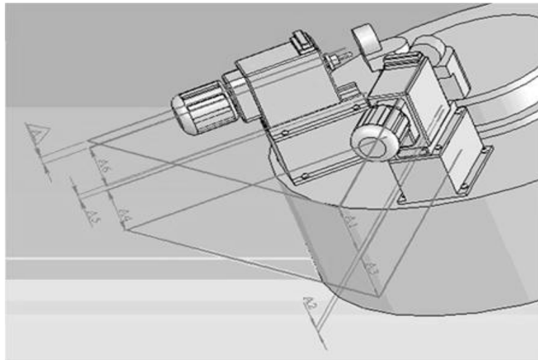
Рис. 6. Модель размерной цепи А, определяющая смещение осей шпинделів на первой и второй позициях обработки.
