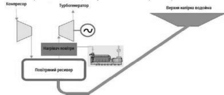
Мал.1 Схема гібридної акумулюючої електростанції
