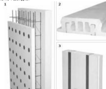
Рис.1 Конструктивні елементи системи PLASTBAU (ПЛАСТБАУ):
