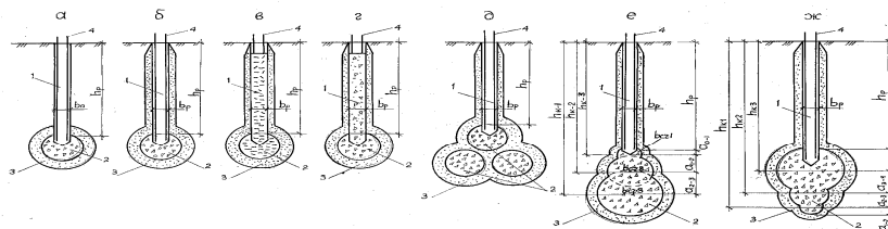
Рис. 1. Конструкции фундаментов в пробитых скважинах с уширением
