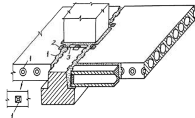
Рис.1. Фрагменти дисків перекриттів зв'язевого каркаса серії 1.020-1 / 83. пустотних плит; 1 - переривчаста шпонка; 2 - закладні деталі; 3 - накладки.
