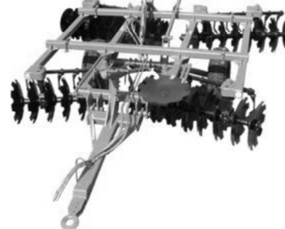
Рис. 1 – Серійна дискова важка борона БДВ-3
