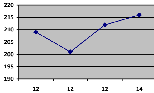
Рис.3: Відношення водонепроникності до міцності бетону (кубики, що просоченні мазутом)
