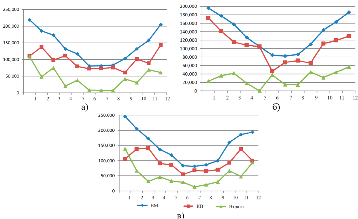
Рис. 1. – Залежності щомісячного відпуску в мережу (ВМ), корисного відпуску (КВ) та втрат для фідера 86-06: а) – за 2022 рік; б) – за 2021 рік; в) – за 2020 рік
