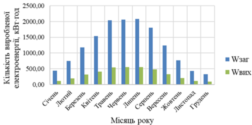
Рис. 2. Річна генерація електроенергії сонячної електростанції
