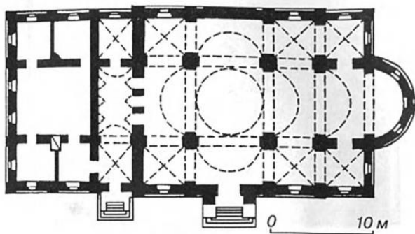
Рис.9. Церква Різдва Іоана Предтечі Мовчанського монастиря. План
