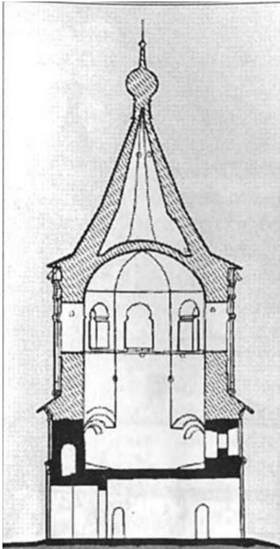
Рис.8. Дзвіниця Мовчанського монастиря. Поздовжній розріз. Креслення В. Вечерського
