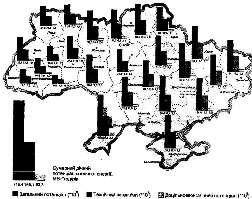
Рис. 13.4. Потенціал сонячної енергії в Україні
