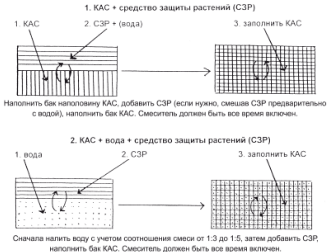
Рис. 57 Приготування робочого розчину при комбінації КАС та засобу захисту рослин
