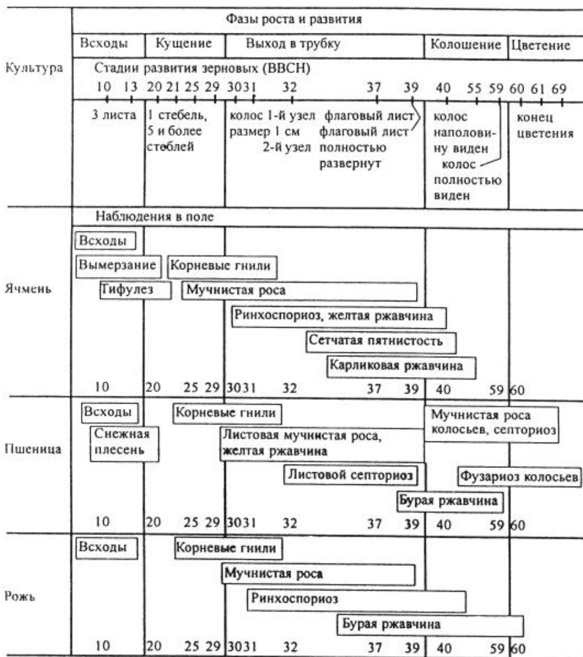
Рис. 61 Терміни спостережень і обліку хвороб у посівах зернових у Німеччині
