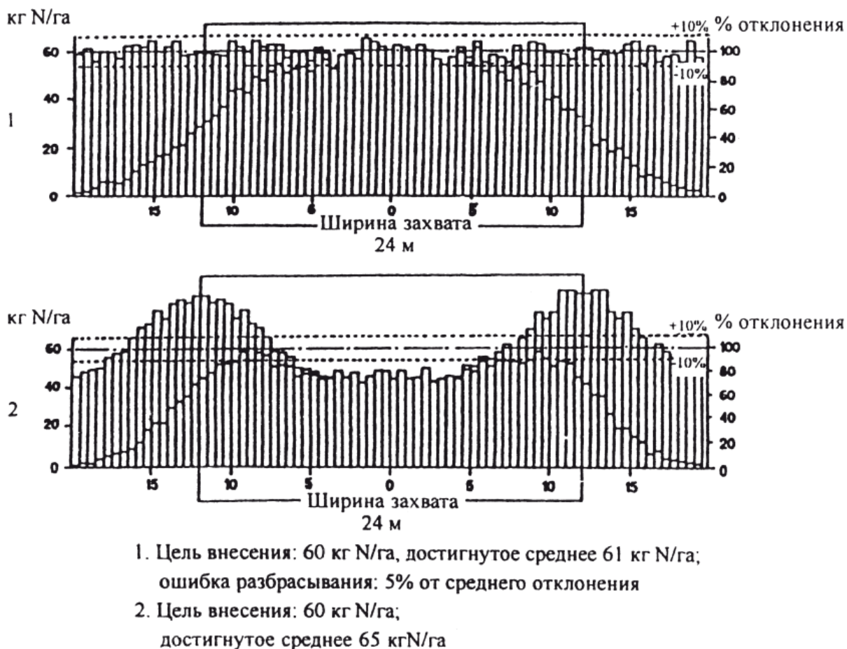
Рис. 44 Точність розкидання азотних добрив при оптимальному розподілі часток (1) і поганій якості (2)
