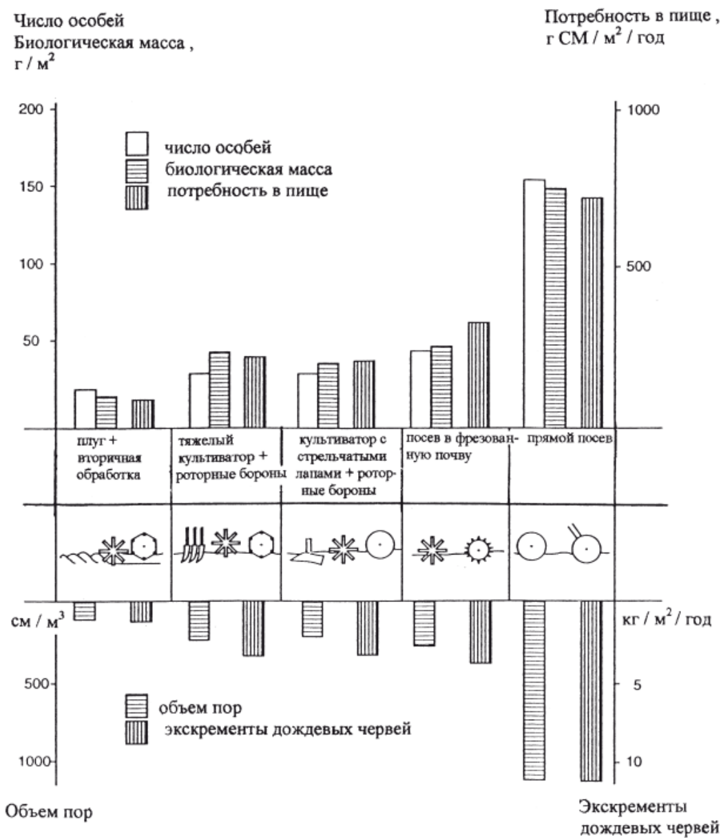
Рис. 18 Кількість дощових черв'яків, накопичення їх біологічної маси, потреба в їжі, обсяг пір і маса їх екскрементів при різних способах обробки ґрунту
