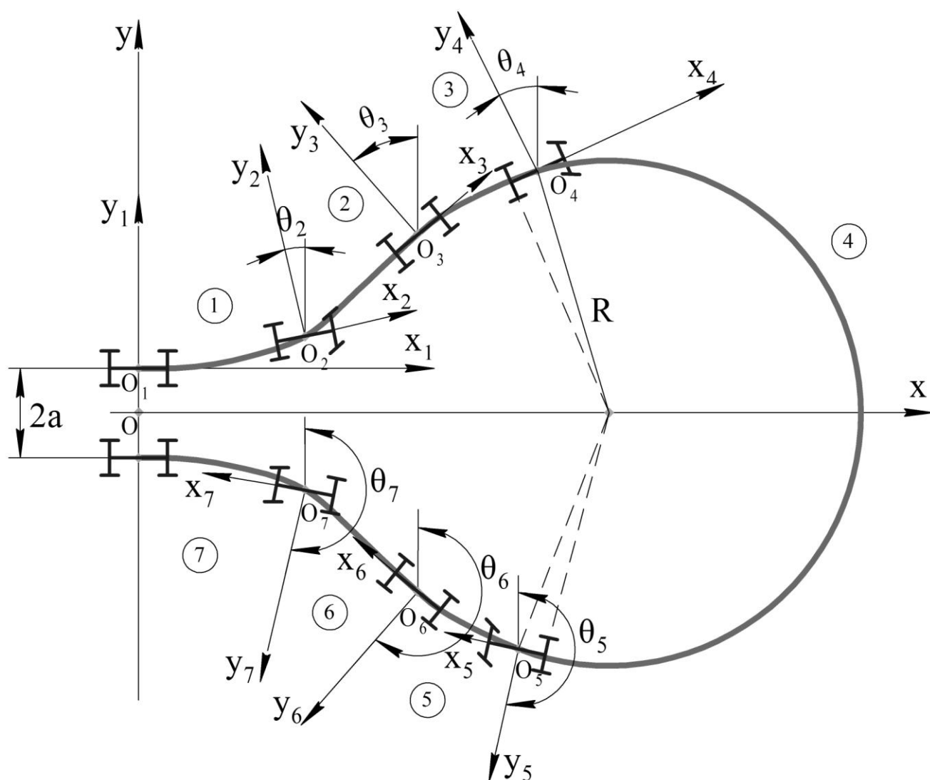
Рисунок 3.1 – Ділянки петлевидного розвороту трактора МТЗ-80 з культиватором КРН-4,2
