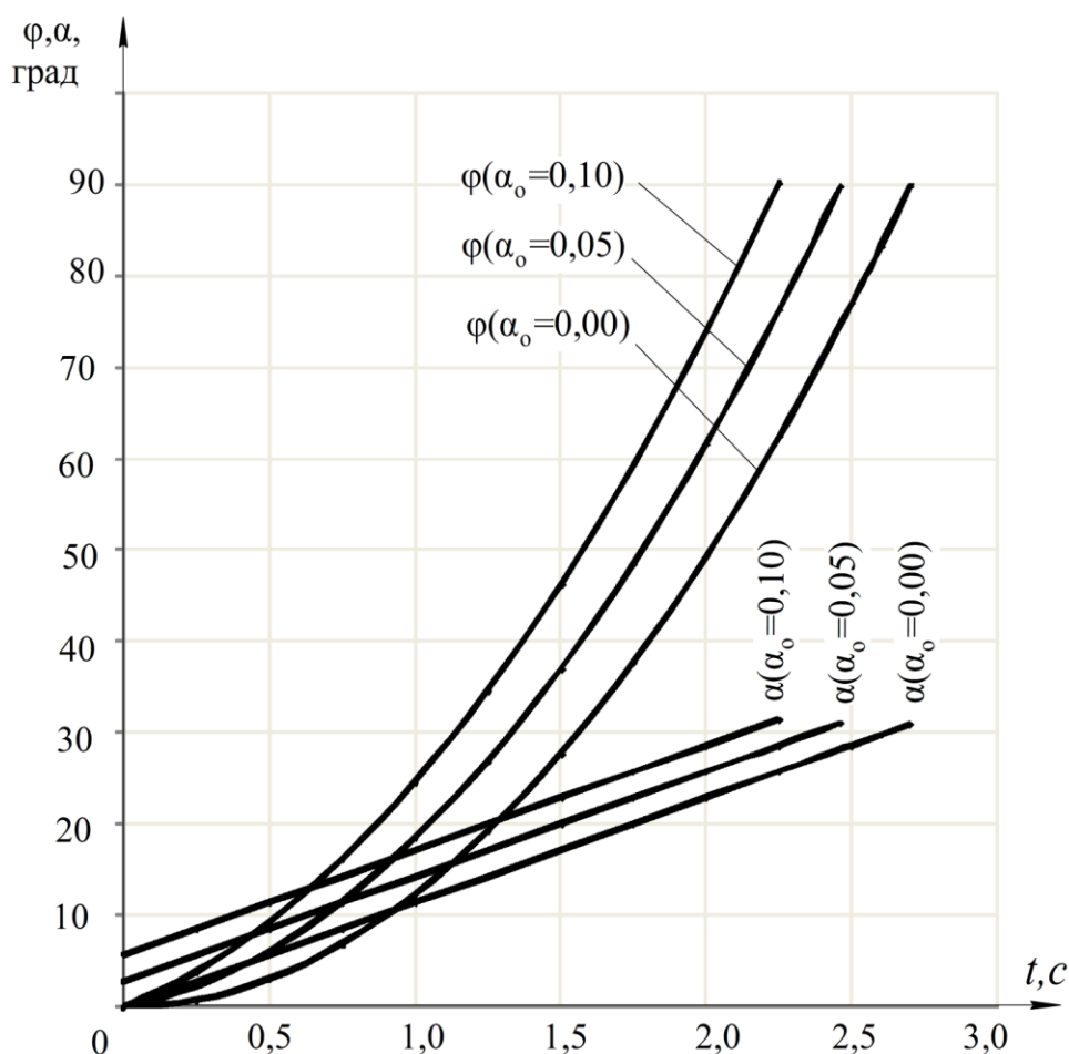
Рисунок 2.19 – Графіки зміни курсового кута \alpha і кута повороту корпусу машини \varphi при різних значеннях \alpha_o , якщо \alpha = \alpha_o + kt ( k = 0,2 \text{ c}^{-1} ; v = 2 \text{ м/с} ; \ell = 0,93 \text{ м} )
