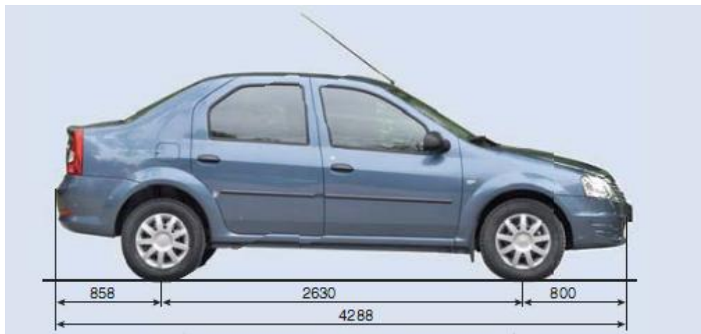
Рисунок 3.6 – Габаритні розміри Renault Logan
