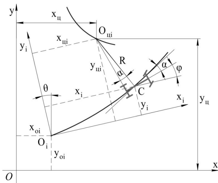
Рисунок 2.25 – До визначення координат лінії миттєвих центрів кривизни траєкторії входу в поворот
