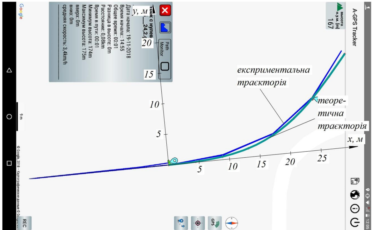
Рисунок 4.12 – Експериментальна та теоретична траєкторії входу в лівий поворот і виходу з лівого повороту чотирьохколісної машини
