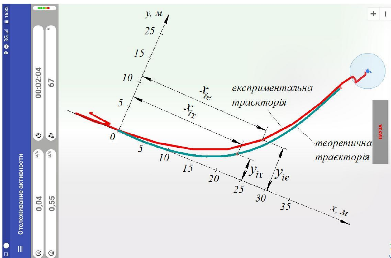
Рисунок 4.14 – Експериментальна та теоретична траєкторії входу в лівий поворот і виходу з лівого повороту чотирьохколійної машини
