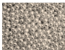
перлини
