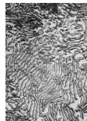
пластинчастий перлит
