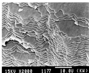
структура перлини
