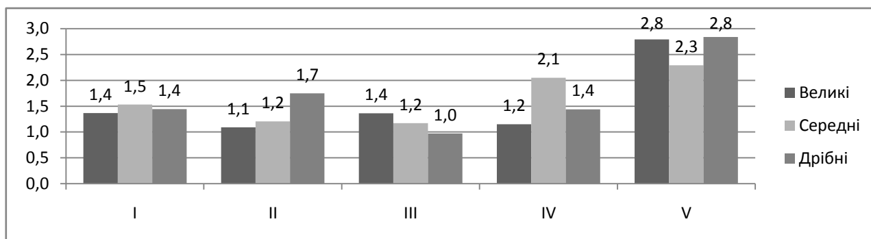
Рис.1. Групи сортів за рівнем середньомісячних втрат бульбами різного розміру в %
