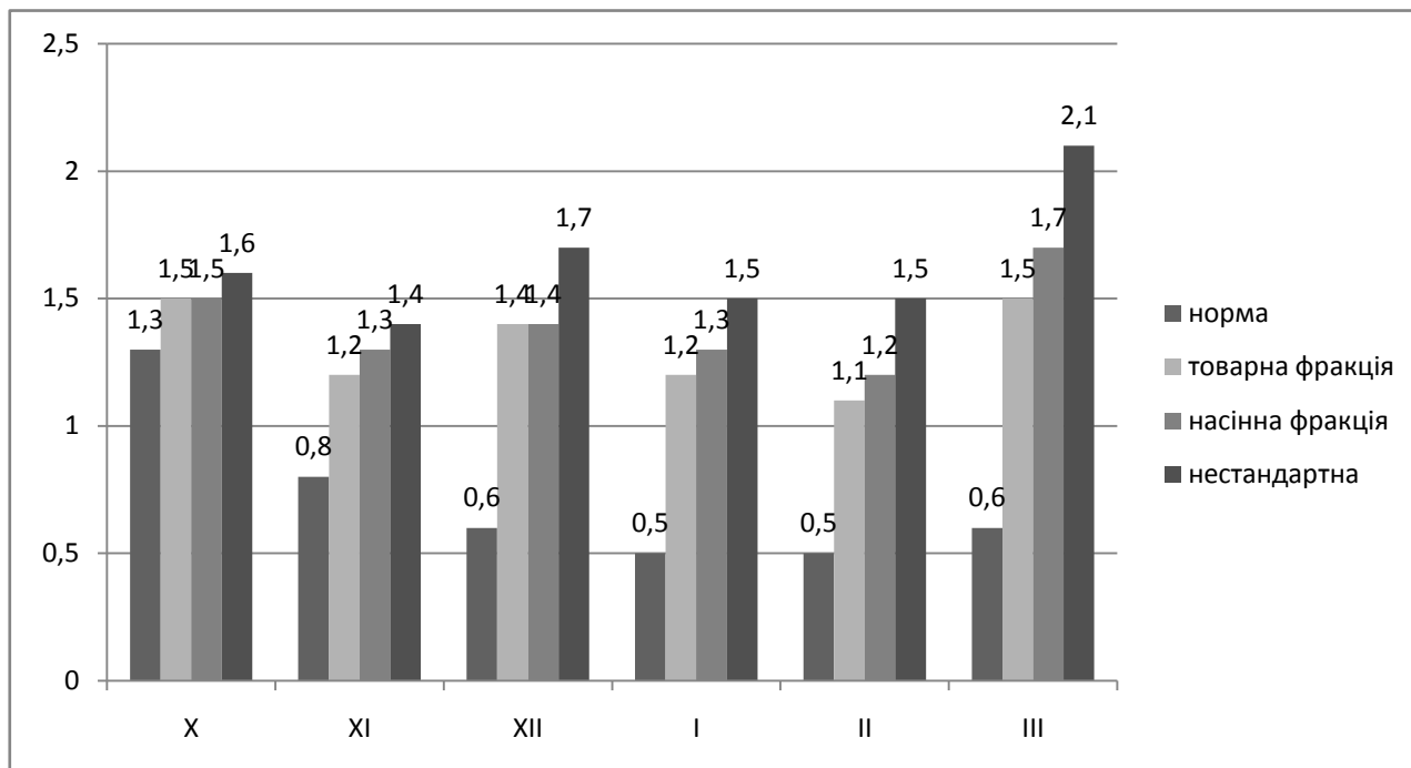
Рис.2. Щомісячні природні втрати сортів картоплі за фракційним складом бульб в %
