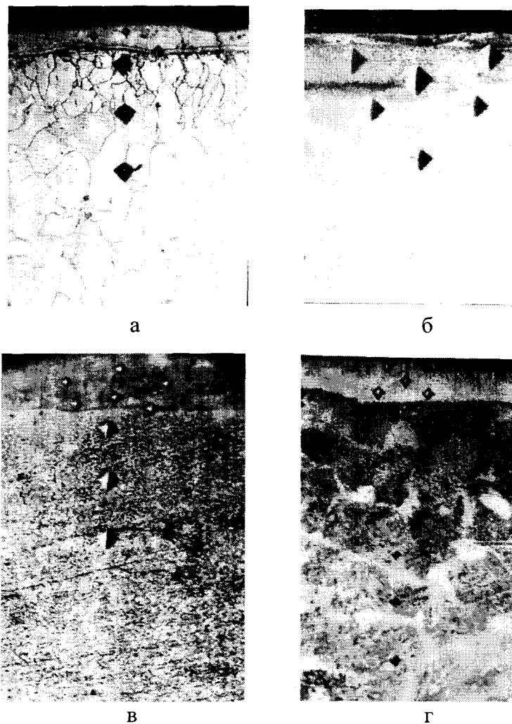
Рис.2 - Микроструктура поверхностного слоя образцов после ЦЭЭЛ а – армко-железо, х 250, нагрузка P=0,02 Н; б - сталь 12Х18Н10Т х 400, нагрузка P=0,05 Н; в – сталь 30Х13 х 400, нагрузка P=0,02 Н; г - сталь 40Х х 200, нагрузка P=0,05 Н.
