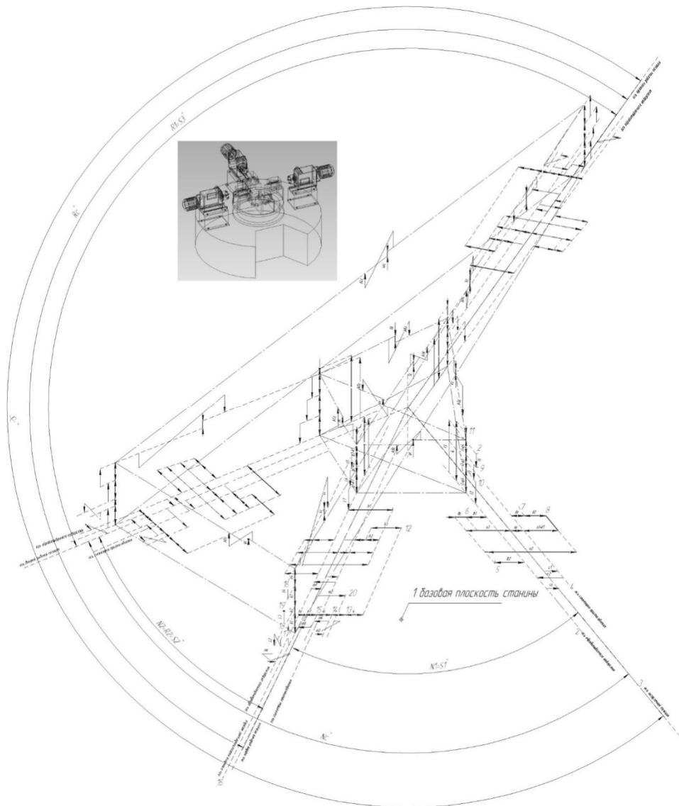
Рис. 1. Тривимірний модель багатопозиційного металорізального верстата і просторові розмірні ланцюги до неї.
