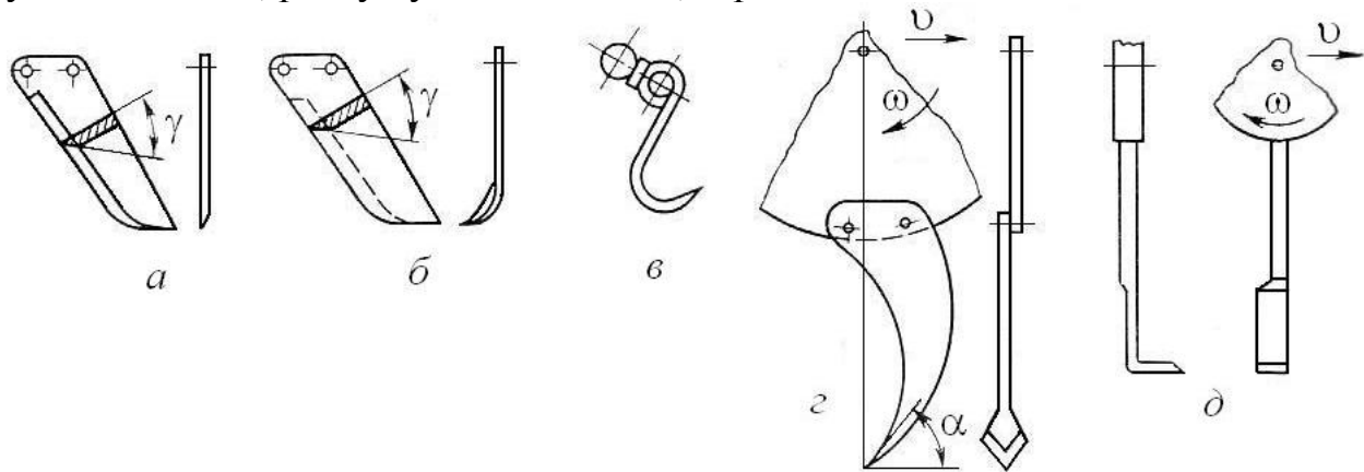
Рис. Основні типи робочих органів фрез і проріджувачів: а – прямий ніж; б – зігнутий ніж; в – пружинний гачок; г – розпушувальне долото; д – ніж проріджувача
