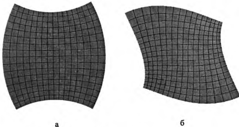
Рис. 1. Відсіки мінімальних поверхонь, побудованих за рівняннями (9): а) при \alpha = 0 ; \beta = 1 ; б) при \alpha = 1 ; \beta = 1
