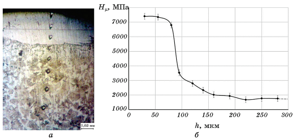
Рис. 4. Микроструктура ( a ) и распределение микротвёрдости в поверхностном слое ( б ) для образца из стали 40X после алитирования методом ЭЭЛ при W_p = 6,8 Дж.
