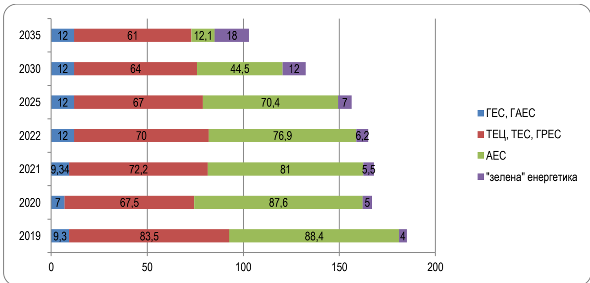
Рис.3. - Прогноз потужностей української енергетики до 2035 року, млрд.кВт-год
