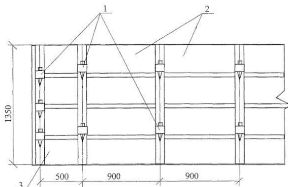
Рис. 3.4 - схема з'єднання щитів опалубки
