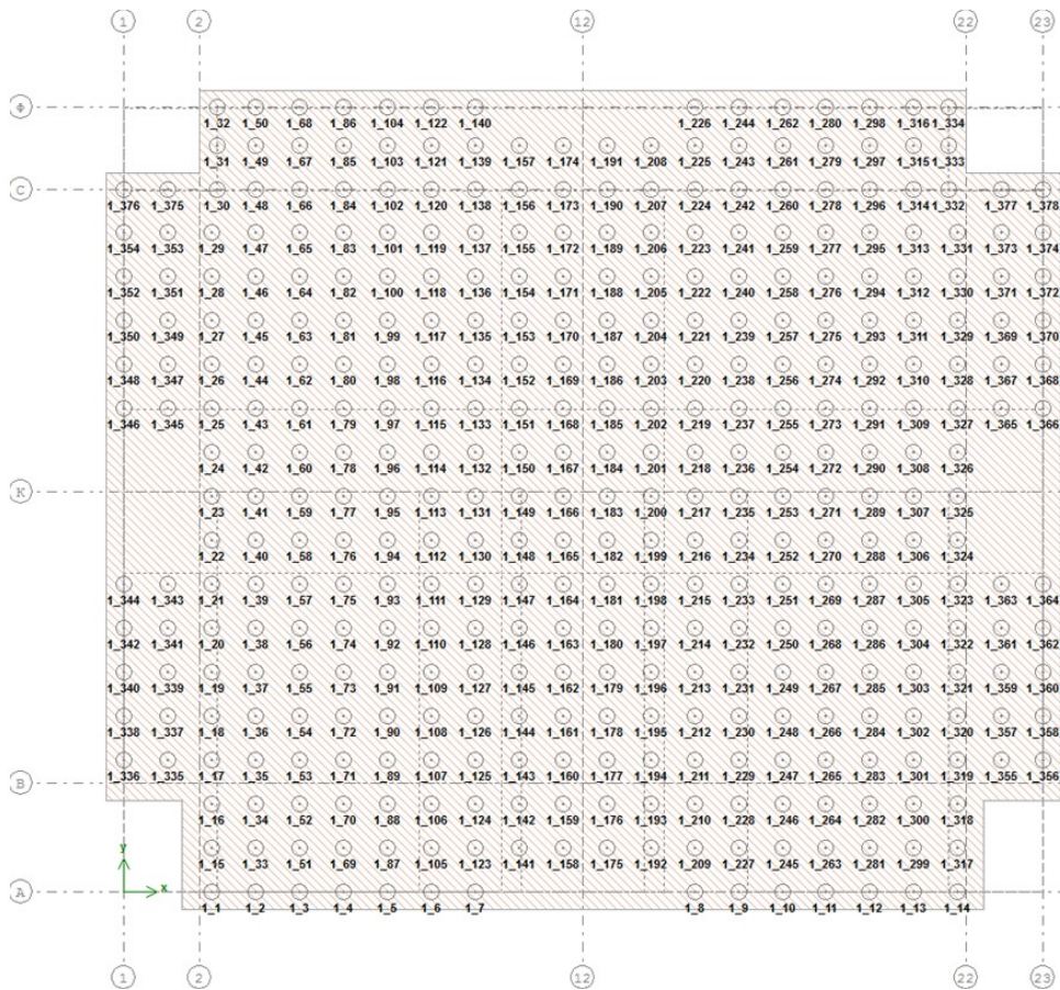
Рис. 2.2. Схема розташування залізобетонних палей довжиною l=6\text{м.}
