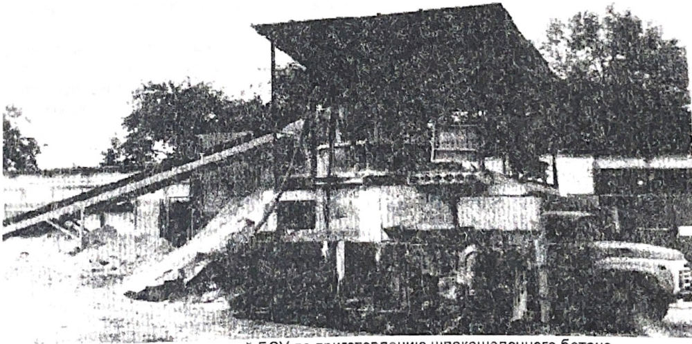
Рис.2. Сезонний БСУ з виготовлення шлаколужного бетону в змішувачі примусової дії V = 1000\text{л} .
