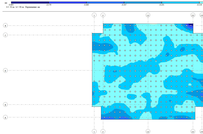
Рис.2.12. Схема осідання монолітної плити розтверку S=0,695\text{м}
