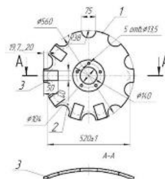
Рисунок 3 – Схема відновлення диску: 1 – новий диск; 2 – зношений; 3 – вставка
