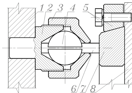
Рисунок 1 Утримувач зразка:
