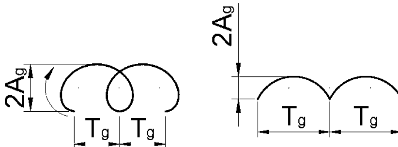
Рисунок 1. Нові форми канавок частково регулярних мікрорельєфів
