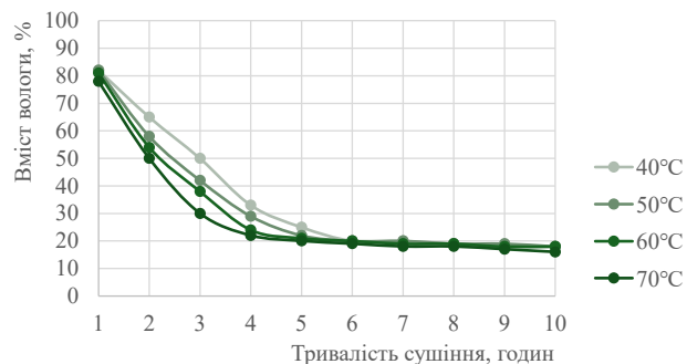
б) інфрачервоне сушіння
