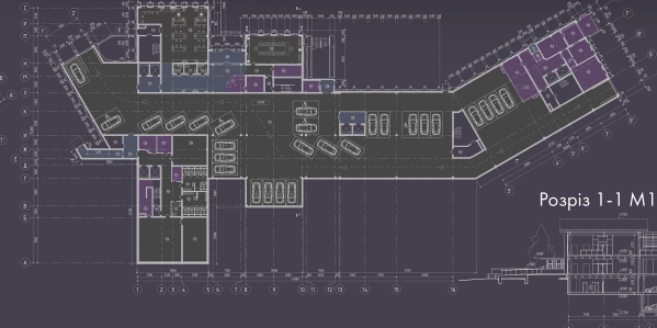
План поверху на відмітці -8.000 М 1:200
