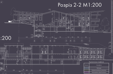
Розріз 2-2 М1:200
