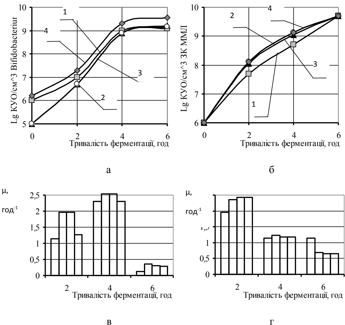
Рис. 2. Зміна мікробіологічних показників: зміна кількості життєздатних клітин монокультур Bifidobacterium (а) та змішаних культур мезофільних
