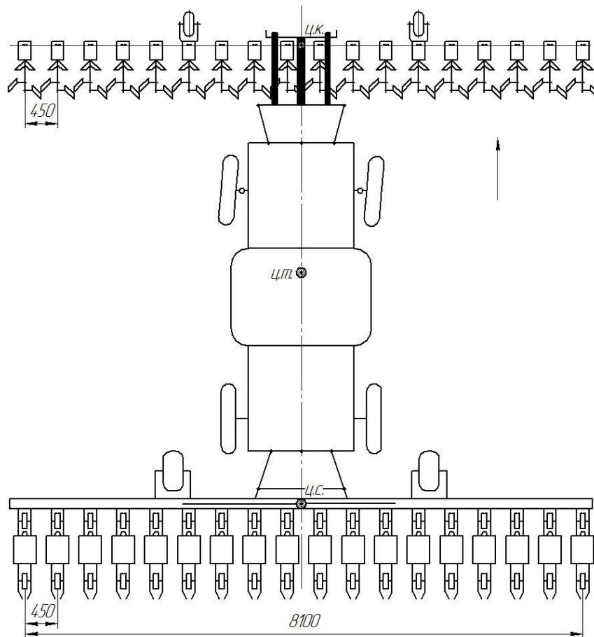
Рис. 1. Схема комбінованого агрегату
