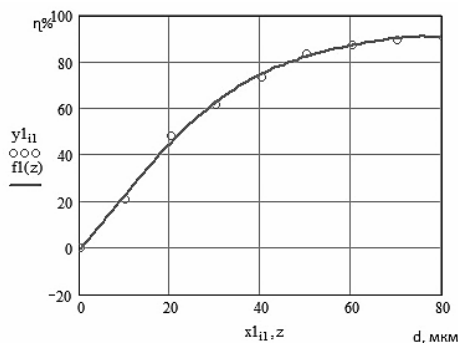
Рис. 3. Інтегральна функція розподілення для АЗПІ до вдосконалення
