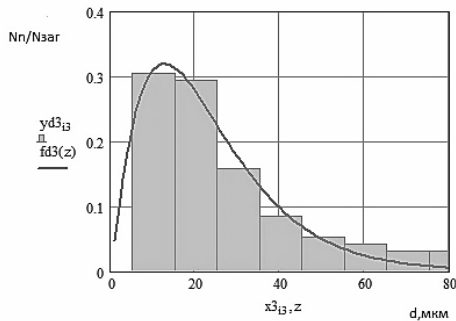
Рис. 8. Диференціальна функція розподілення на тлі експериментальної дискретної гістограми, яка вказує на кількість частинок різних розмірів (АЗЗП після вдосконалення з одним конусом)
