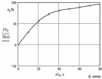
Рис. 7. Інтегральна функція розподілення для АЗЗП після вдосконалення (з одним конусом)
