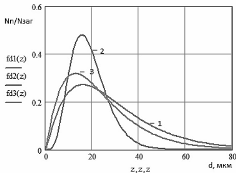
Рис. 10. Диференціальні функції розподілення для трьох апаратів із зустрічними закрученими потоками: 1 – АЗЗП до вдосконалення; 2 – АЗЗП після вдосконалення (із двома конусами); 3 – АЗЗП після удосконалення (із одним конусом)
