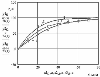
Рис. 9. Інтегральні функції розподілення для трьох апаратів із зустрічними закрученими потоками: 1 – АЗЗП до вдосконалення; 2 – АЗЗП після вдосконалення (із двома конусами); 3 – АЗЗП після удосконалення (із одним конусом)
