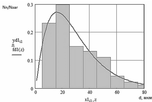
Рис. 4. Диференціальна функція розподілення на тлі експериментальної дискретної гістограми, яка вказує на кількість частинок різних розмірів (АЗПІ до вдосконалення)
