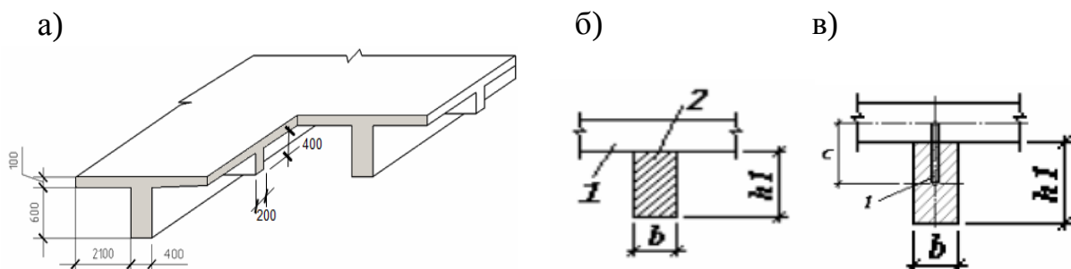
Рис.2 Фрагмент ребристого перекриття (а); розміщення стержня відносно плити (б); ексцентриситет стиків в вузлах елементів (в).
