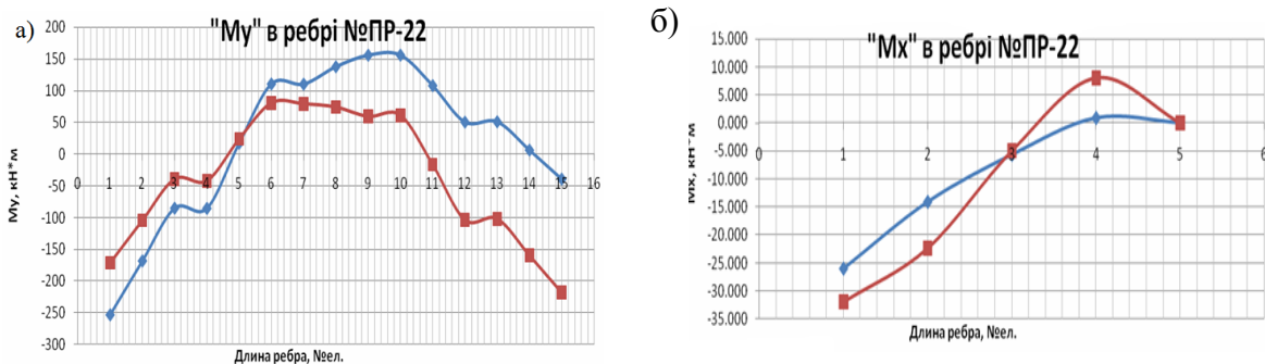
Рис. 4. Епюри згинальних моментів (а) та крутних моментів (б) в ребрі №22 для пружного розрахунку і для розрахунку з урахуванням нормальних тріщин; — — пружний розрахунок; — розрахунок при змінених жорсткостях при крученні та при згині.
