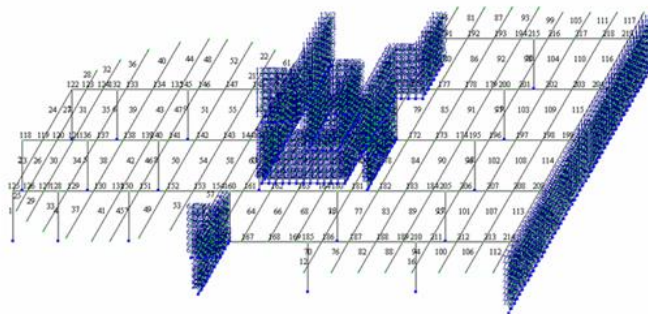
Рис.3 Фізична модель фрагменту монолітного ребристого перекриття (а), розрахункова схема монолітного перекриття (б)
