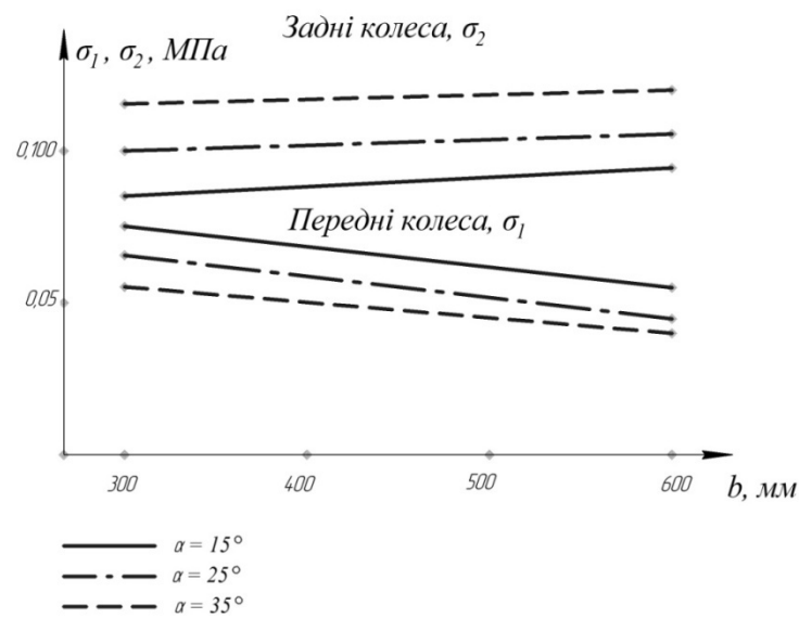
Рисунок 3 – Залежність напружень в ґрунті від висоти крюка
