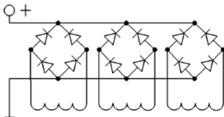
Обмотки статора генератора
