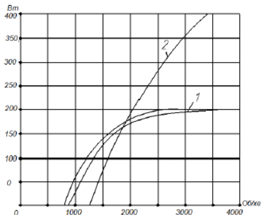
Рисунок 2 – Графік залежності потужності генераторів (1 – стандартні, 2- підвищеної потужності)
