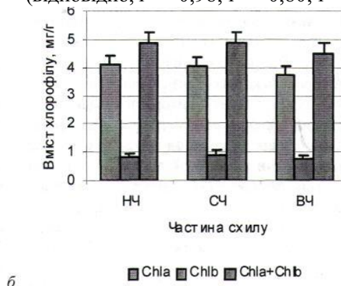
Рис. 1. Вміст хлорофілу а (Chla), хлорофілу b (Chlb) та сумарний вміст (Chla+Chlb) у листках A. platanoides (а) і R. pseudoacacia (б) у природній діброві на нижній (НЧ), середній (СЧ) і верхній (ВЧ) частинах правобережного схилу р. Самара
