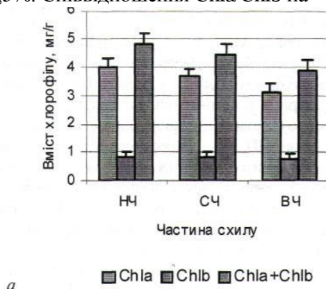
Рис. 1. Вміст хлорофілу а (Chla), хлорофілу b (Chlb) та сумарний вміст (Chla+Chlb) у листках A. platanoides (а) і R. pseudoacacia (б) у природній діброві на нижній (НЧ), середній (СЧ) і верхній (ВЧ) частинах правобережного схилу р. Самара
