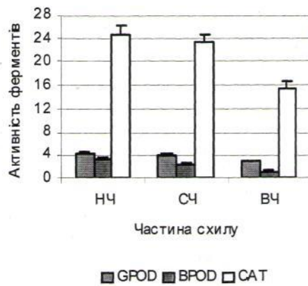
Рис. 2. Активність гваякол-пероксидази (GPOD, мМ тетрагваяколу/г*хв), бензидин-пероксидази (BPOD, опт. од./г-хв), каталази (CAT, мкМ H 2 O 2 /г-хв) у листках A. platanoides (а) і R. pseudoacacia (б) у природній діброві на нижній (НЧ), середній (СЧ) і верхній (ВЧ) частинах правобережного схилу р. Самара
