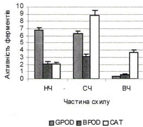
Рис. 2. Активність гваякол-пероксидази (GPOD, мМ тетрагваяколу/г*хв), бензидин-пероксидази (BPOD, опт. од./г-хв), каталази (CAT, мкМ H 2 O 2 /г-хв) у листках A. platanoides (а) і R. pseudoacacia (б) у природній діброві на нижній (НЧ), середній (СЧ) і верхній (ВЧ) частинах правобережного схилу р. Самара
