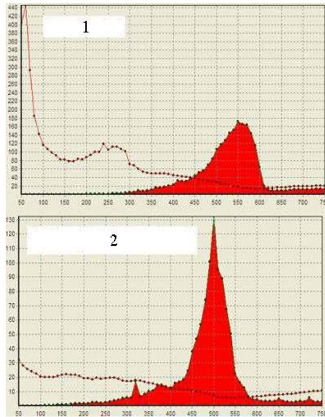
Рис. 6. Термограми іонів \text{CO}_2 , отриманих з бетонних зразків, модифікованих добавкою на основі жовтого залізоокисного пігменту та контрольного зразка: вісь ординат – Signal intensity, a.u.; вісь абсцис – температура; 1 – Cement (control); 2 – Cement + iron oxide yellow pigment \text{Fe}(\text{OH})\text{O} , \text{FeNO}_2 , 1 %
