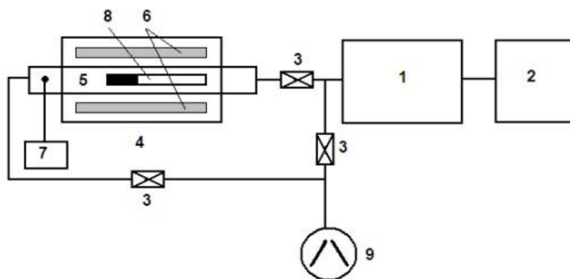
Рис. 1. Установка термопрограмованої мас-спектрометрії (ТПД-МС): 1 – мас-спектрометр; 2 – ПК; 3 – вакуумні крани; 4 – піч (1200 °С); 5 – вакуумована кварцова трубка; 6 – нагрівальні елементи; 7 – термопара; 8 – кварцова пробірка зі зразком; 9 – турбомолекулярний насос
