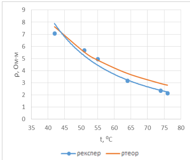
Рисунок 1 – Залежності питомого опору від температури при M_{\text{ном}}^{\text{зр}} = 0,002 кг.
