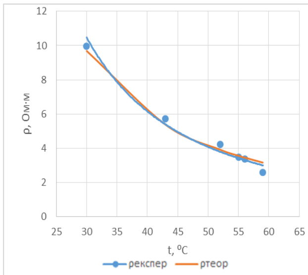
Рисунок 2 – Залежності питомого опору від температури при M_{\text{ном}}^{\text{зр}} = 0,0015 кг.
