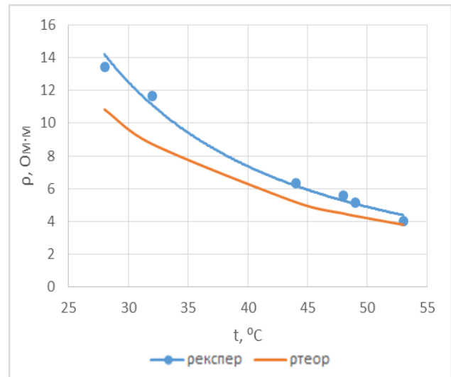
Рисунок 3 – Залежності питомого опору від температури при M_{\text{ном}}^{\text{зр}} = 0,001 кг.
