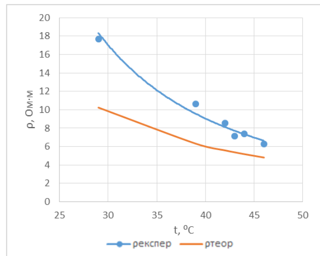
Рисунок 4 – Залежності питомого опору від температури при M_{\text{ном}}^{\text{зр}} = 0,0007 кг.
