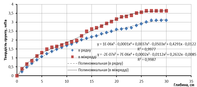
Рис. 10 Твердість ґрунту на плоскорізному обробітку.
