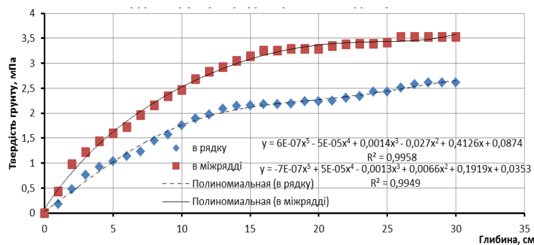
Рис. 11 Твердість ґрунту на дискуванні 12 см.
