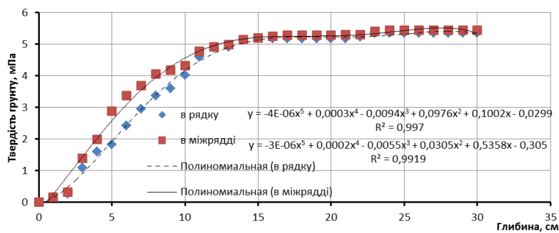
Рис. 6 Твердість ґрунту на на плоскорізному обробітку.
