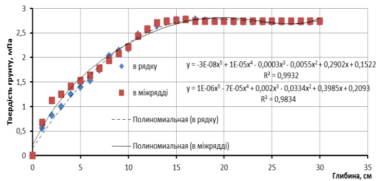
Рис. 3 Твердість ґрунту на дискуванні 12 см.
