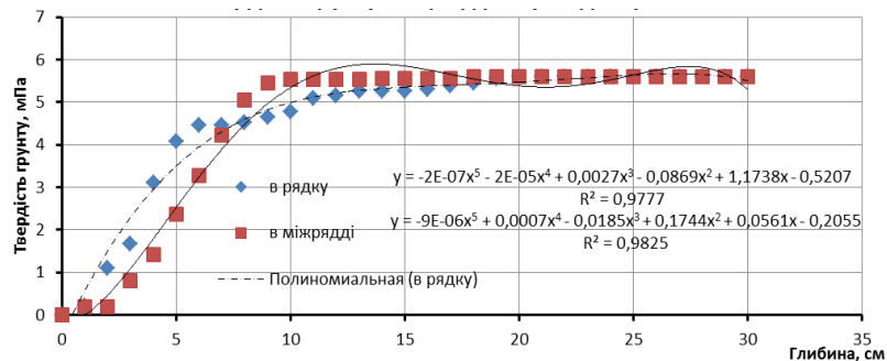
Рис. 7 Твердість ґрунту на дискуванні 12 см.
