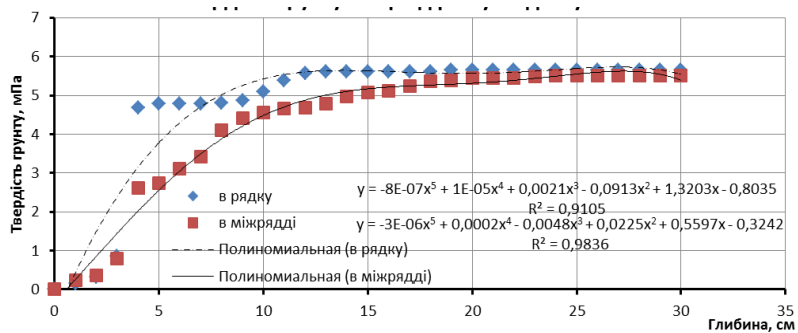
Рис. 8 Твердість ґрунту на дискуванні 6 см.
