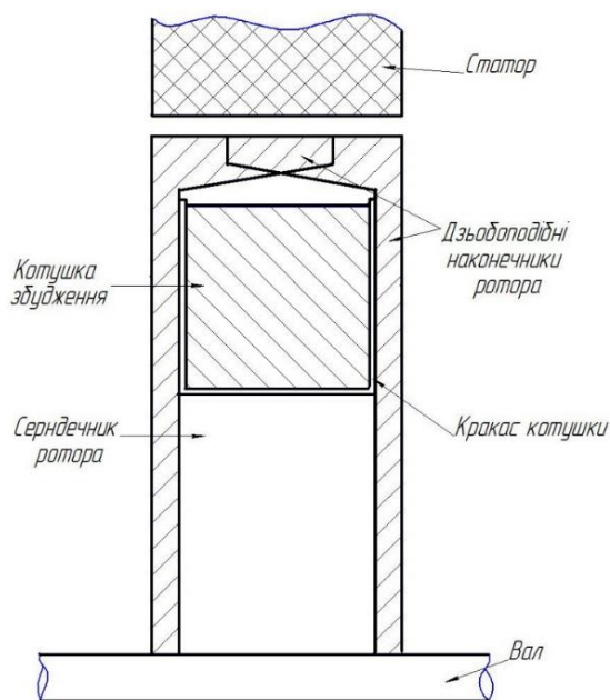
Рис. 4 Магнітний ланцюг генератора для вітросилової установки з дзюбоподібними наконечниками
